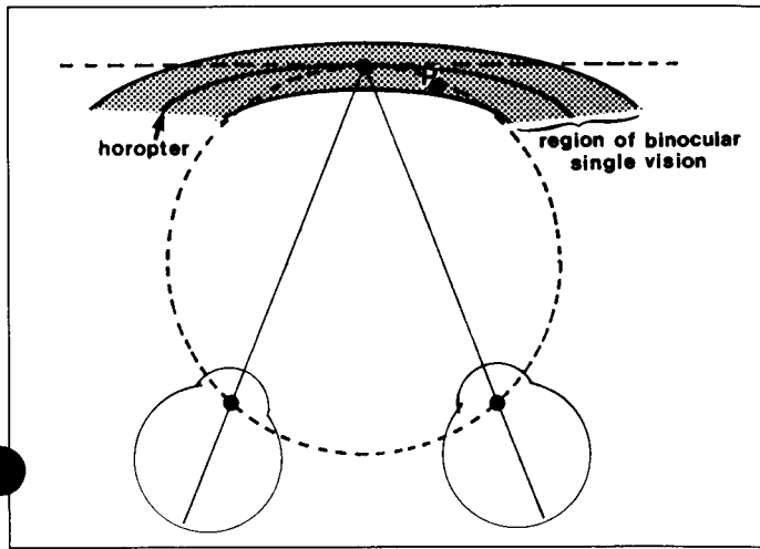
Abb. 3 Horopter und Panumraum, aus [1]
